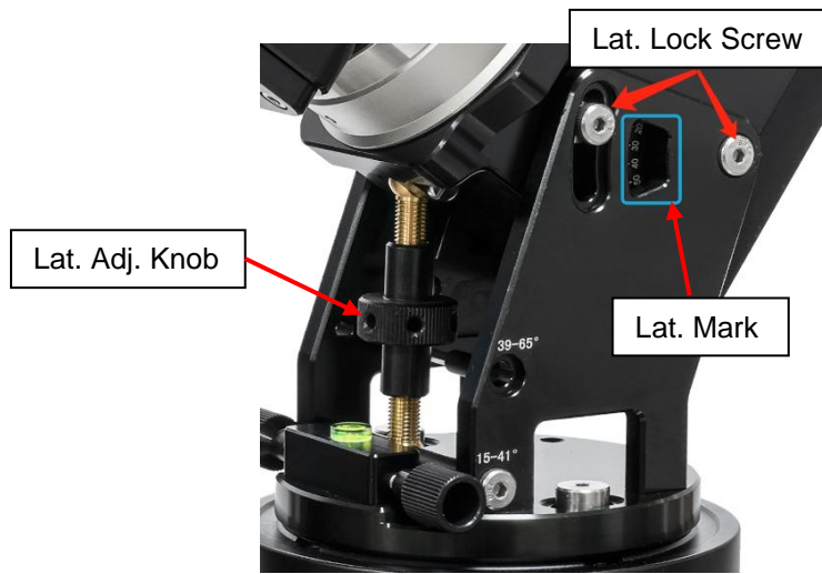
Figure 11. Adjust latitude
